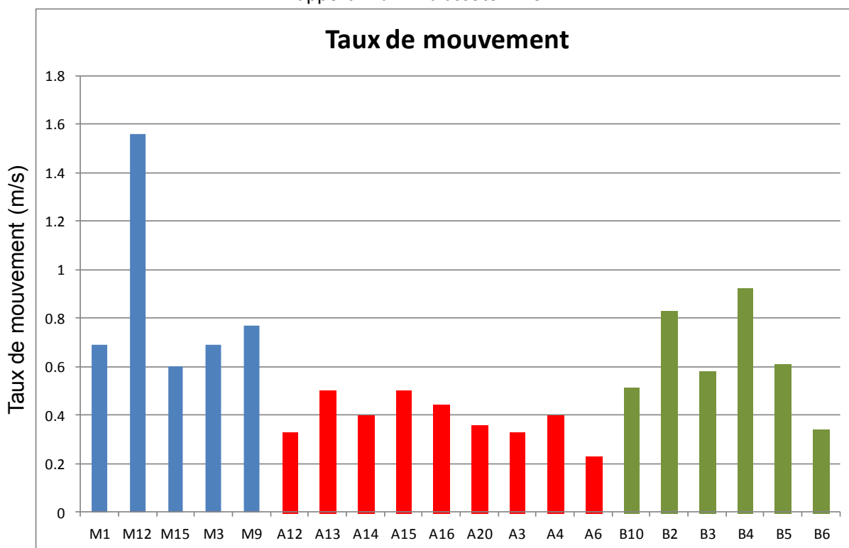
Figure 87 Taux de mouvement moyen (en m/s) par individu calculés à partir des unités de base non fixes de la trajectoire (Distance hydrographique/ \Delta t ).
