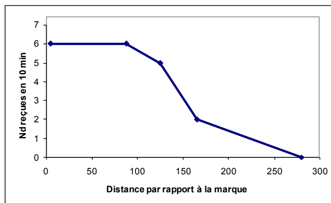
Figure 72 Evolution du nombre de détections d'un émetteur V9 par un récepteur VR2W en fonction de la distance.
