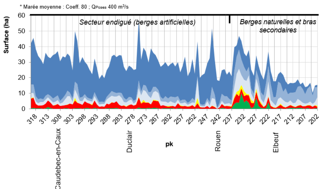
Figure 17. Surface des différents types de milieu le long de la partie fluviale de l'estuaire de la Seine
