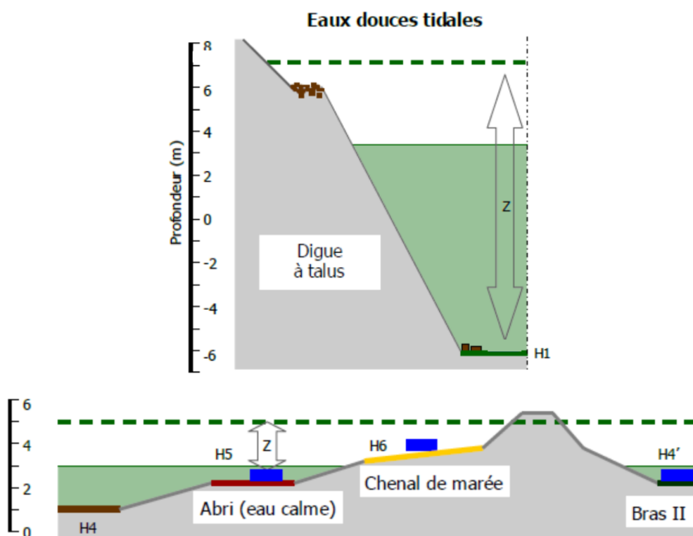
Figure 18. Profils morphologiques schématisés dans le domaine dulçaquicole tidal d'un secteur fortement aménagé (Estuaire de Seine en aval de Rouen, en haut) en comparaison avec un secteur qui l'est moins (amont de Rouen, en bas) (Modifié depuis Duhamel et Feunteun, 2012)
