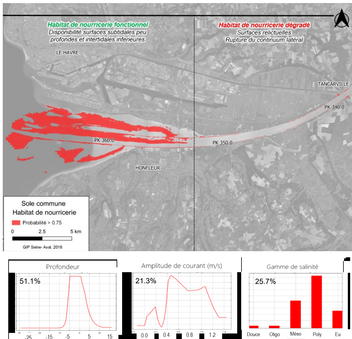
Figure 8. En haut : Distribution des habitats de nourricerie de la sole ( Solea solea ) résultant de la modélisation Maxent. En bas : preferendum écologique pour chaque descripteur, défini sur la base des valeurs qui contribuent davantage à l'assignation des probabilités pour la prédiction des habitats favorables
